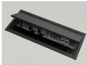
top access with multifunctional sockets passacavi con prese multifunzione
