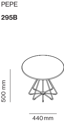
top Ø 500 - 700 mm
