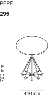
top Ø 500 - 700 mm
