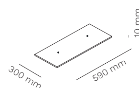
ballast zavorra
