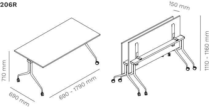
ARGO TILTING table with tilting top tavolo con piano ribaltabile
